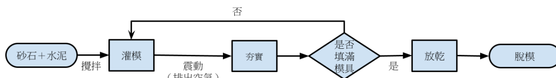
圖一：水泥花格磚製作流程 （圖一資料來源：研究者繪製）
